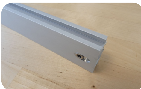
Traverse aluminium anodisé avec pince, LG: 1500 mm ou 600 mm REF/L3GS
