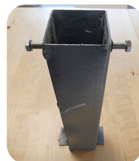
Fourreau acier galva avec 2 serrages boulon Ht: 300 mm REF/FMS5.2
